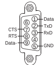
COM3 RS-232/RS-485
